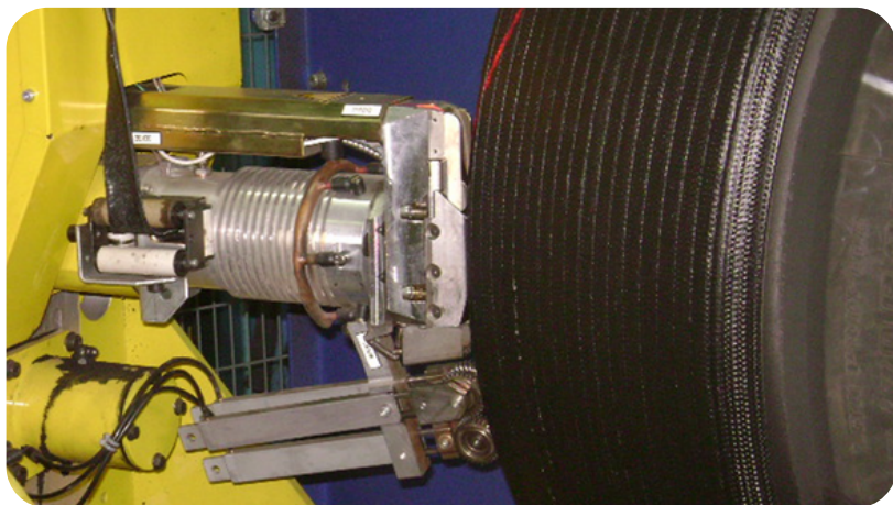
Robotizirani proces nanosa međugume
